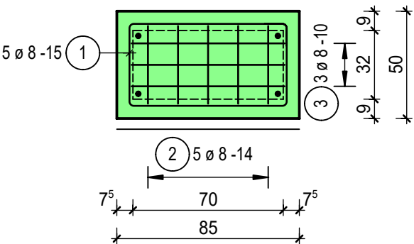
Draufsicht M 1:25
